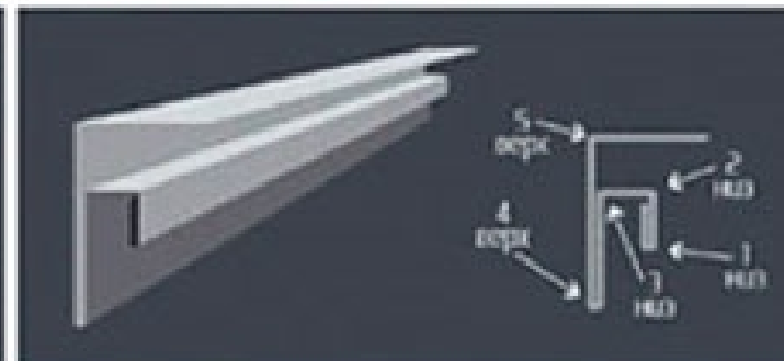
ВНУТРЕННИЙ УГОЛ
