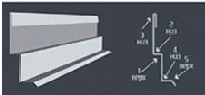
ОБЛИЦОВОЧНЫЙ БОРДЮР
