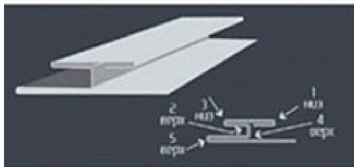
ВЫНОСНОЙ КАРНИЗ
