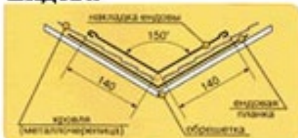
Ендова
