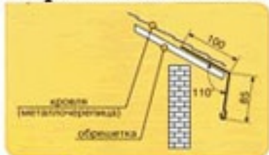
Карнизная планка
