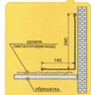
Стыковая планка
