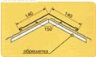
Конек
