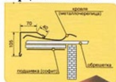
Торцевая планка
