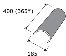
Конек полукруглый одинарный
