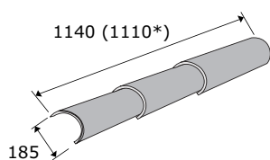
Конек полукруглый тройной
