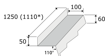
Боковое примыкание (левое, правое)
