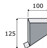
Заглушка торцевой планки ПВХ (левая, правая)
