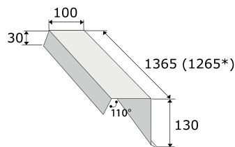
Торцевая планка (универсальная)
