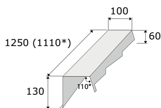
Торцевая планка (левая, правая)
